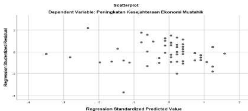
Gambar 1. Uji Heteroskedastisitas
